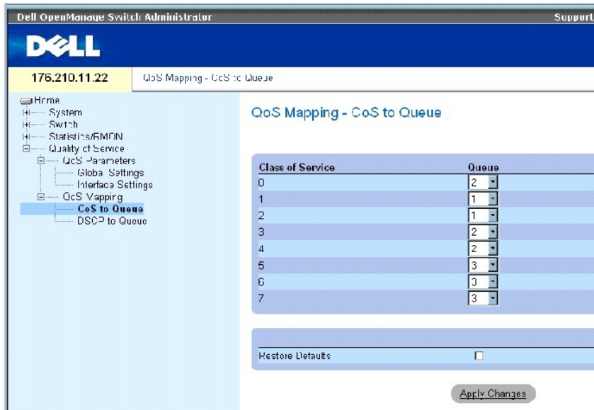
그림 9-3. 대기열의 CoS
